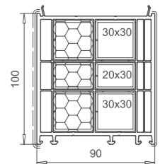
Verbreiterung 100mm 114.207 Stahl 113.025 113.019
