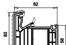
Blendrahmen 83mm Art.-Nr. 101.291 Verstärkungen 113.001 oder 113.367 Haustür
