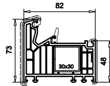
Blendrahmen 73mm Art.-Nr. 101.290 Verstärkungen 113.025 oder 113.365 U-Stahl
