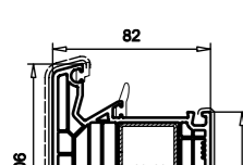
Blendrahmen 106mm Art.-Nr. 101.292 Verstärkungen 113.025 oder 113.365 U-Stahl
