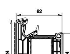
Setzpfosten 124mm Art.-Nr. 102.311 Verstärkungen 113.011 / 1,5mm geschweißt 113.011.2 / 2mm geschweißt 113.011.3 / 3mm geschweißt Verbinderset 106.332 / weiß u. schwarz
